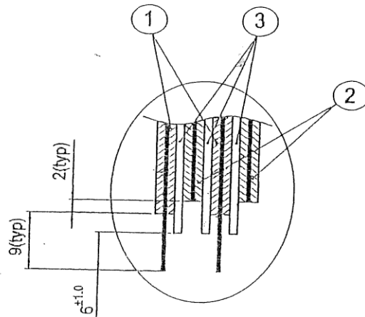
DETAIL-D
