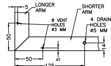
DETAL - "A"
