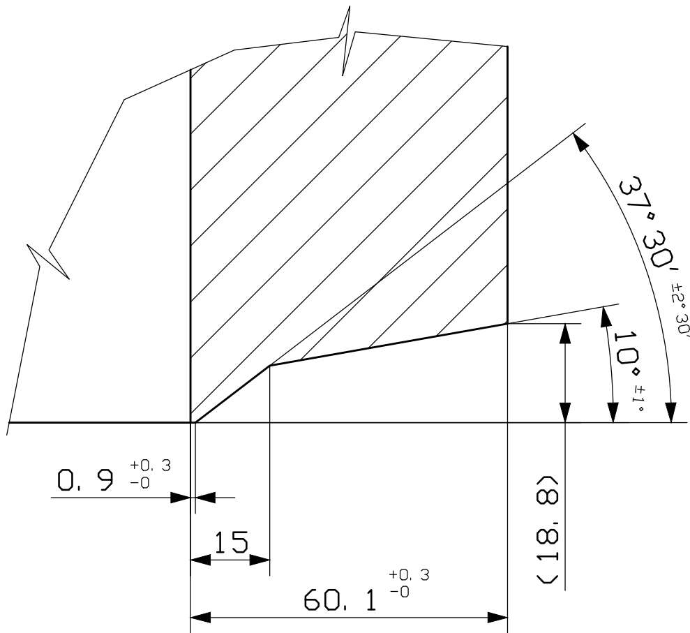
DETAIL-B (1:1)
