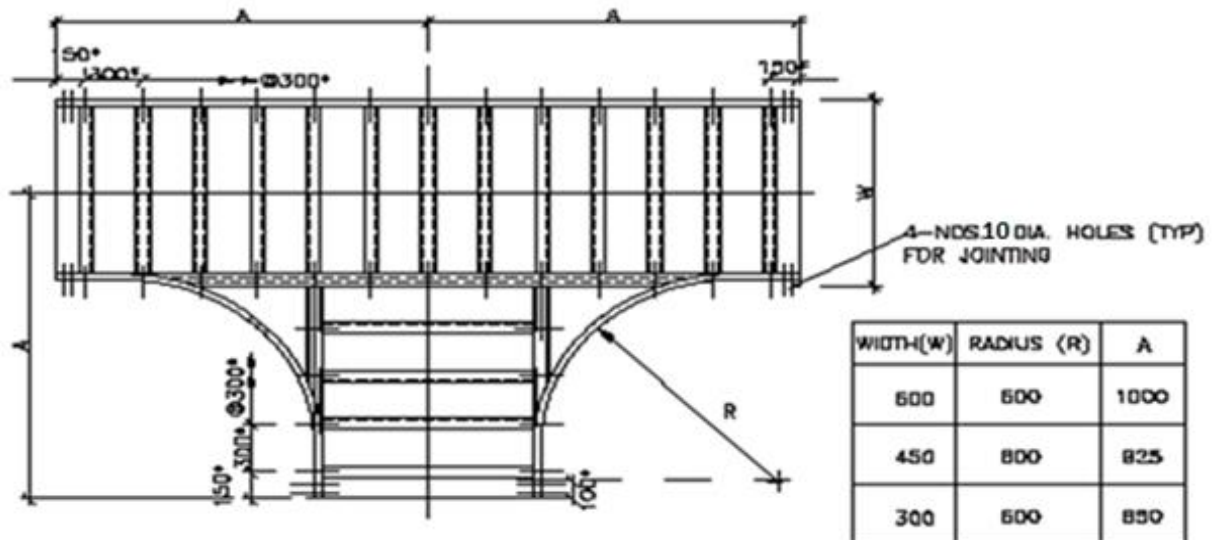
HORIZONTAL TEE-PLAN
