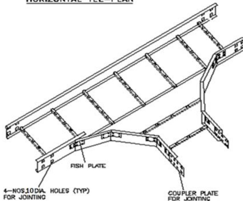
HORIZONTAL TEE
