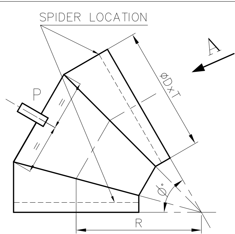
45°/60° MITRE BEND
