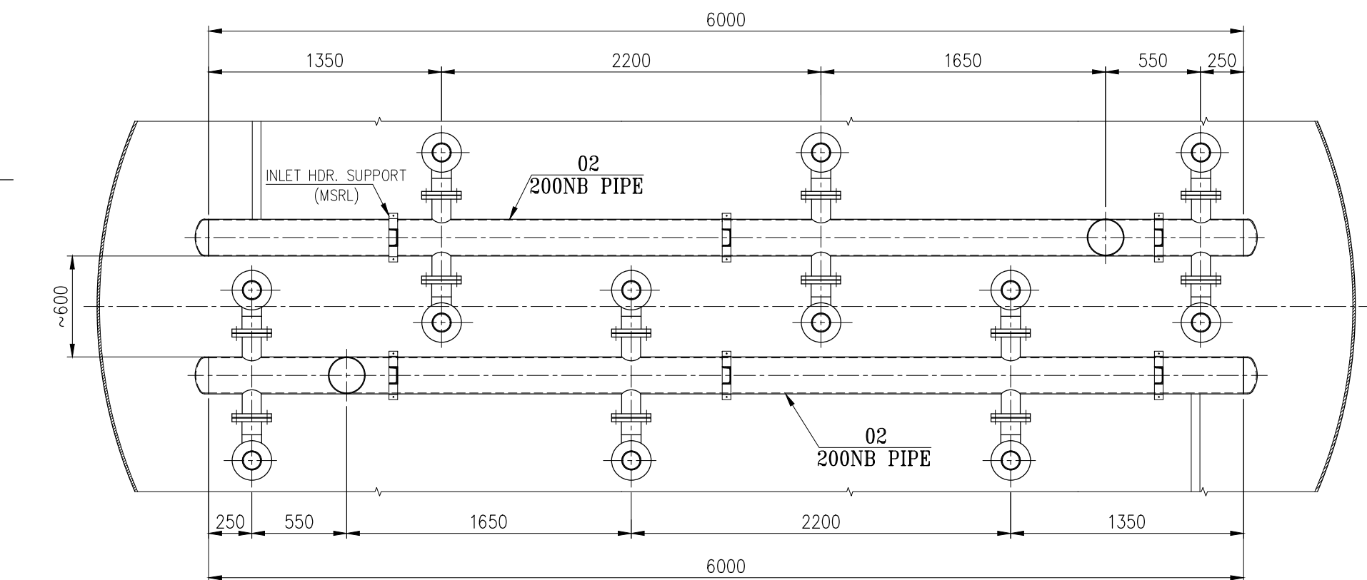
ELEVATION (MEDIA NOT SHOWN)
