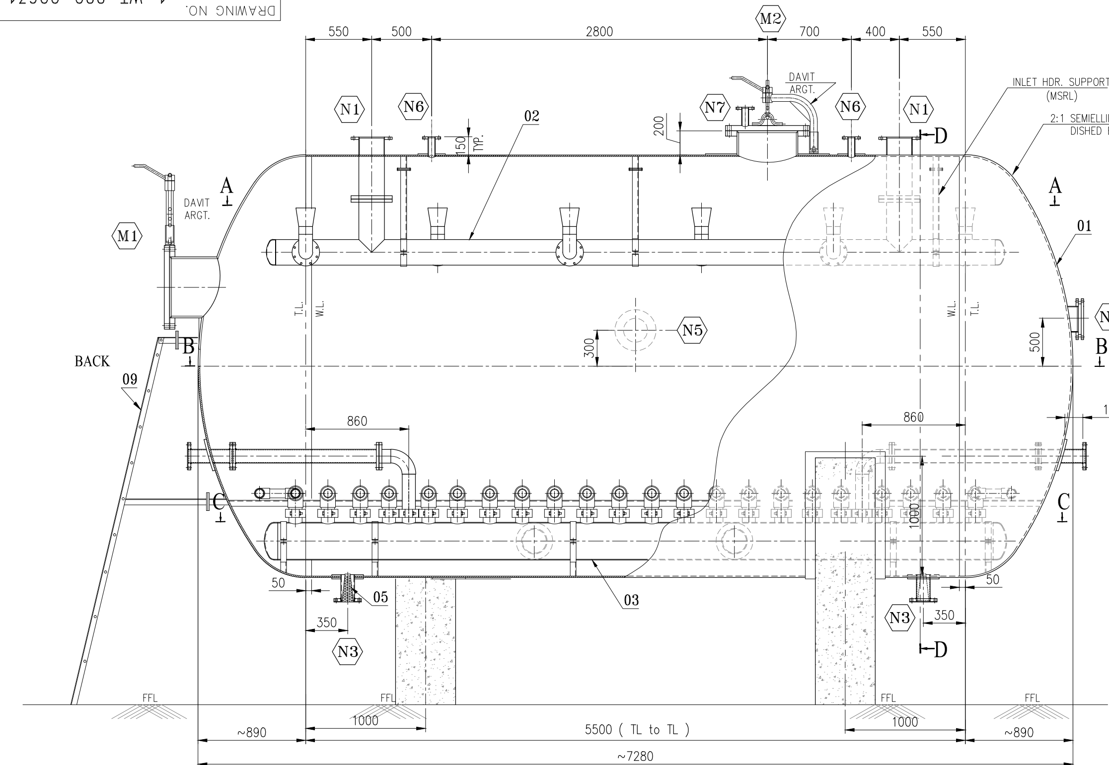
ELEVATION (MEDIA NOT SHOWN)
