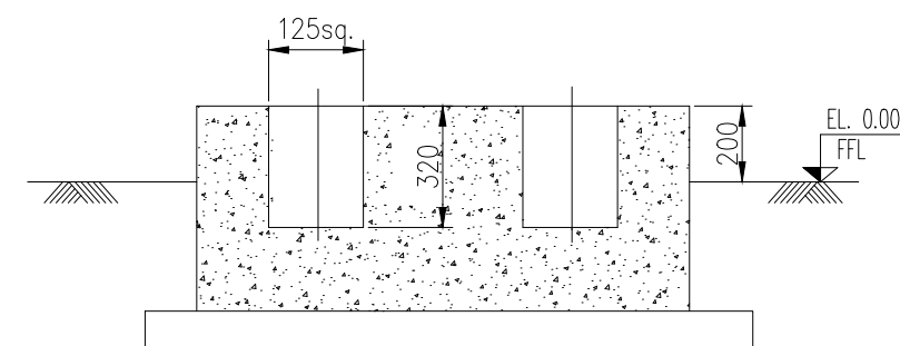
SECTION D-D
