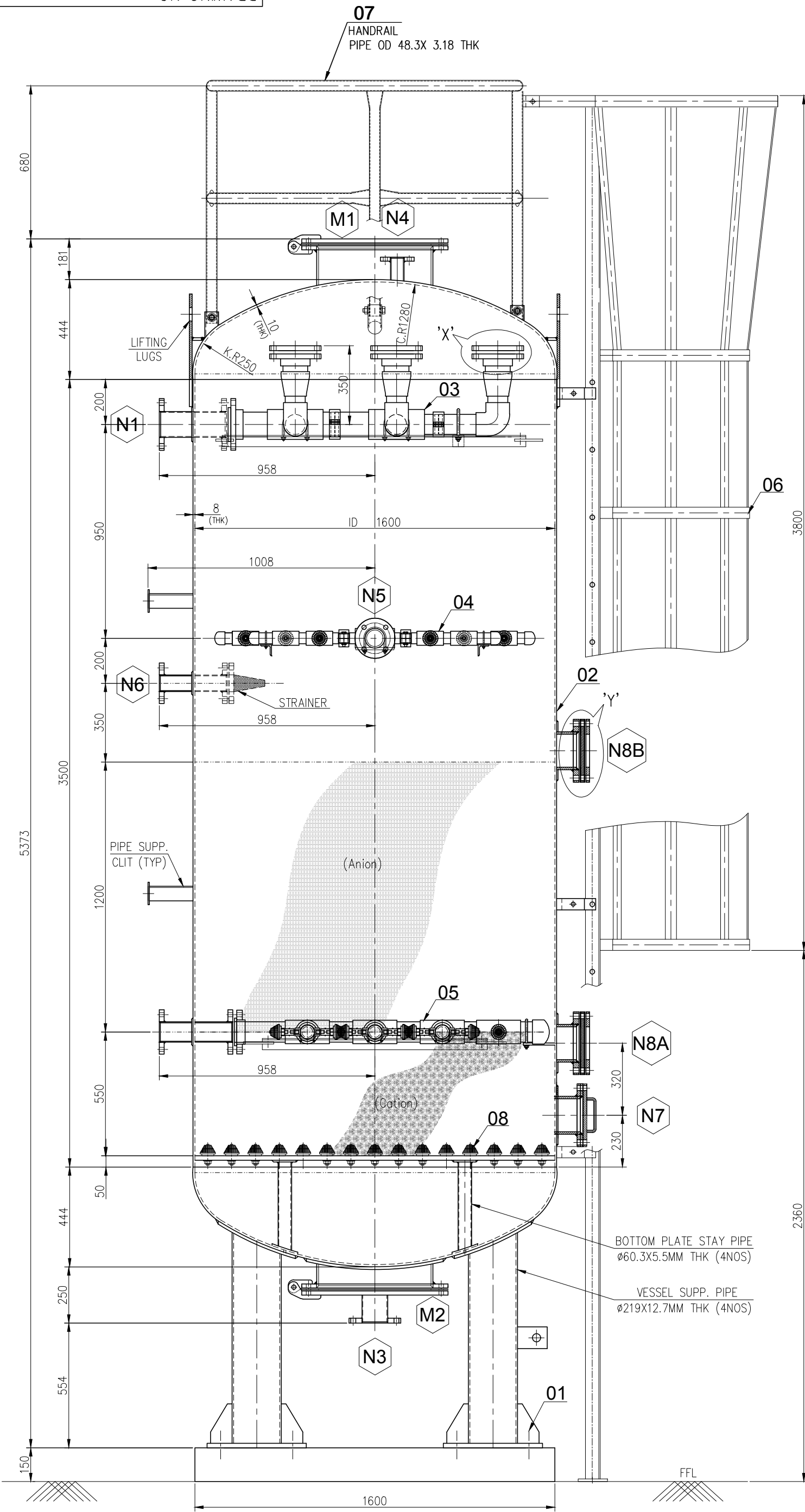
ELEVATION
