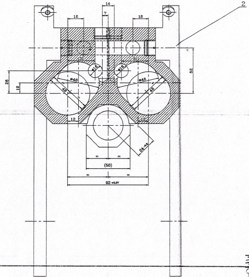
SECTION D-D ZONE L4, J5
