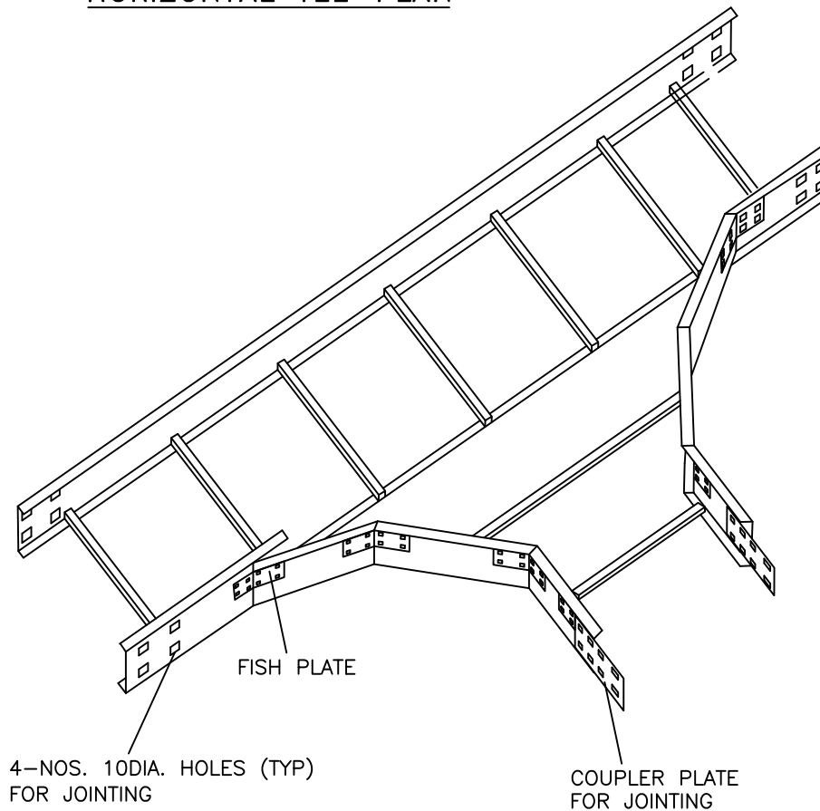
HORIZONTAL TEE
