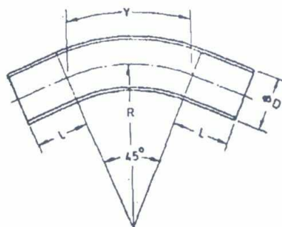
FIG. 1 45° BEND
