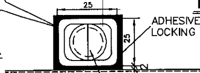
SEC-AA
