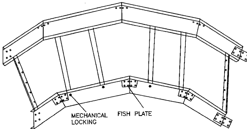
90° HORIZONTAL BEND
