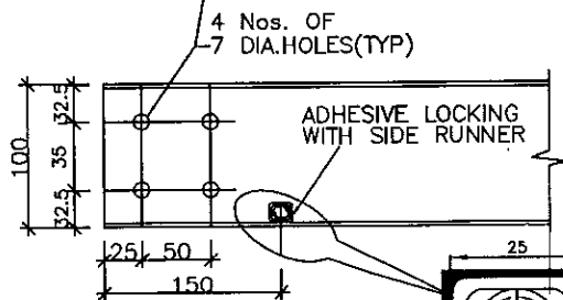
SEC-AA
