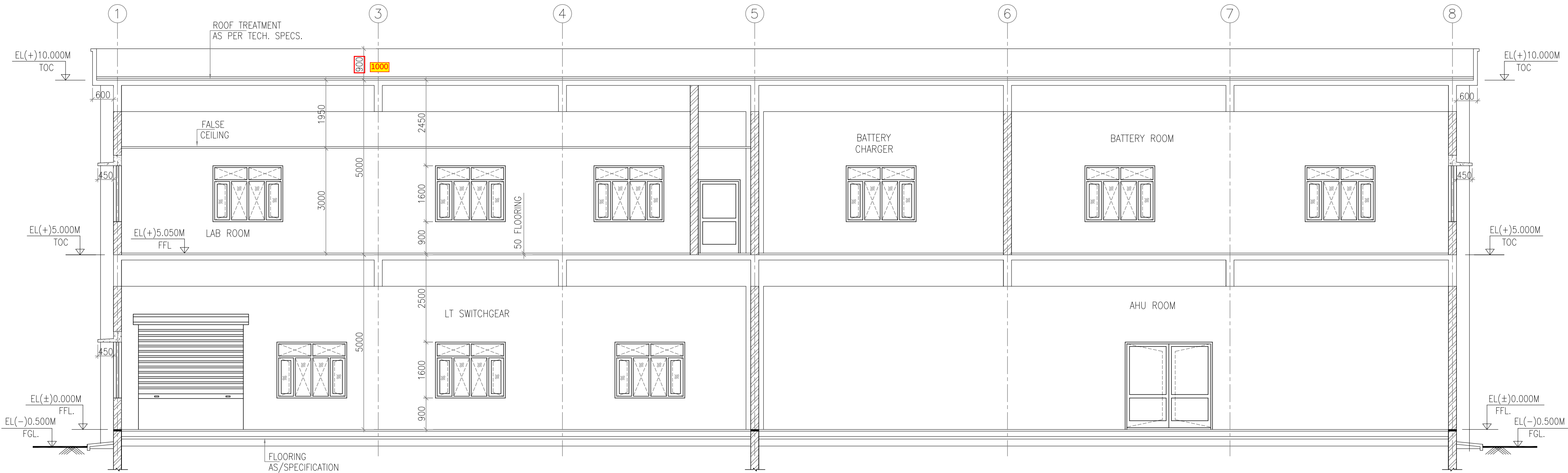
SECTION A-A
