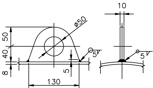
LUG DETAIL-N
