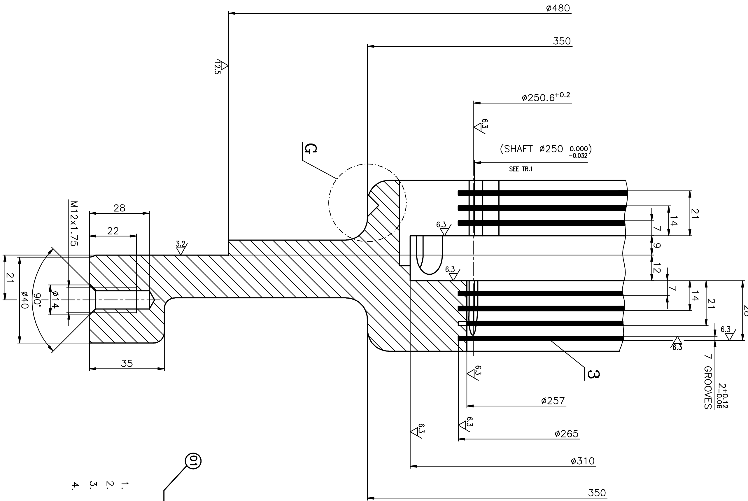
DETAIL-E SCALE 1:1
