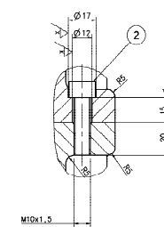
SECTION - D-D (F2)
