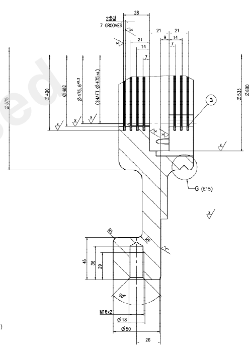
DETAIL - E (J9) 1:1
