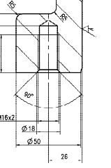
DETAIL - E (J9) 1:1
