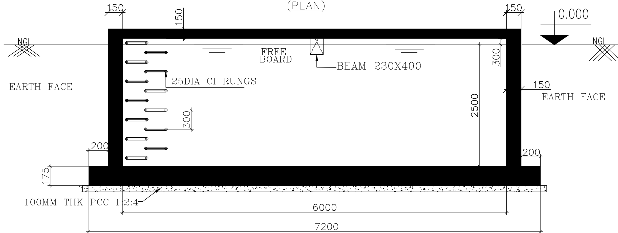
SECTION A-A
