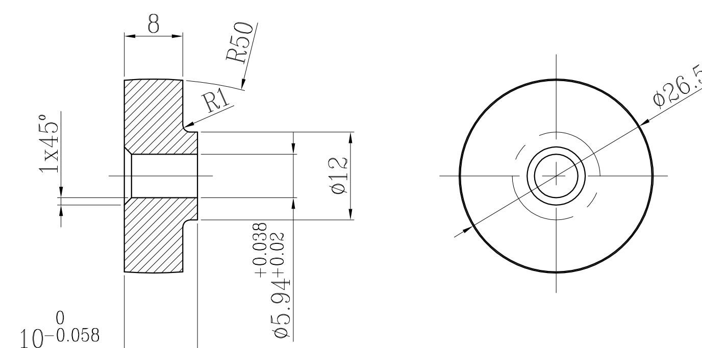
ITEM-13 ROLLER
