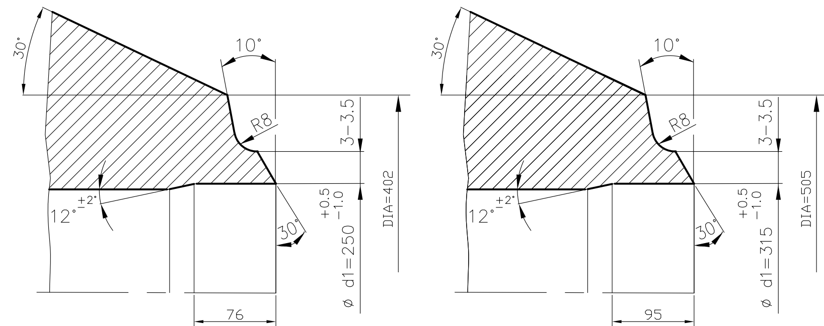
DETAIL-D
