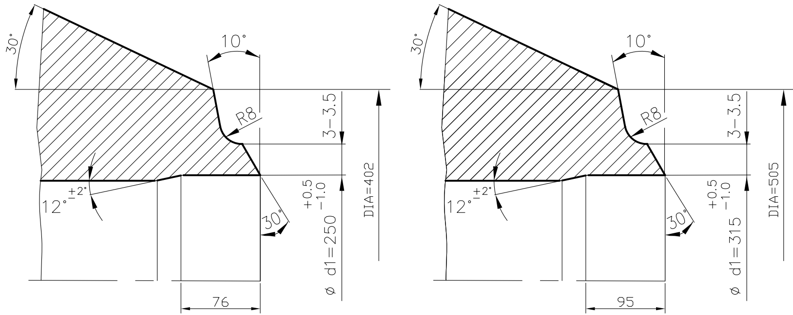
DETAIL-D
