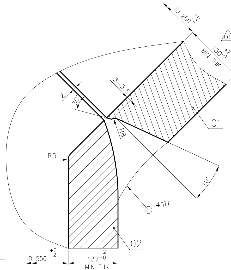
DETAIL-B
