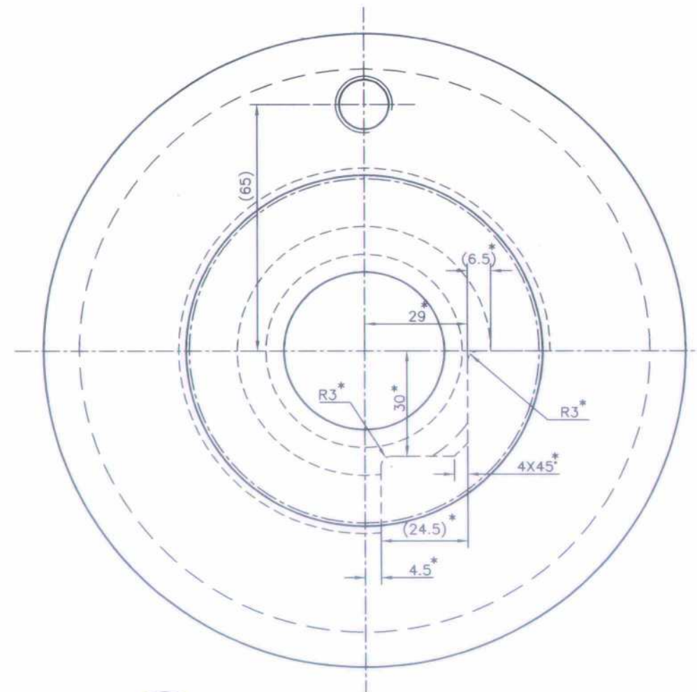
201 TOP DIE
