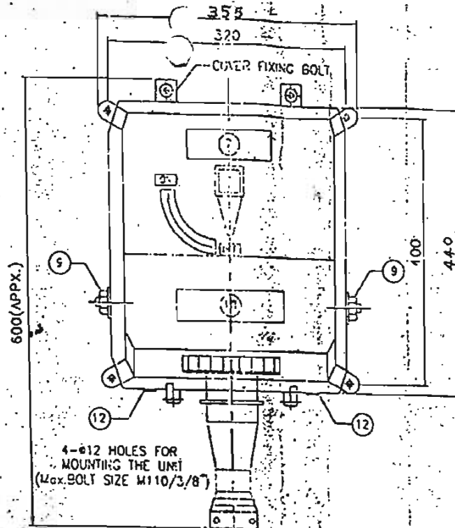
ELEVATION
