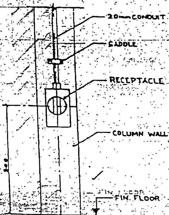
RECEPTACLE - TYPE 'R B '
