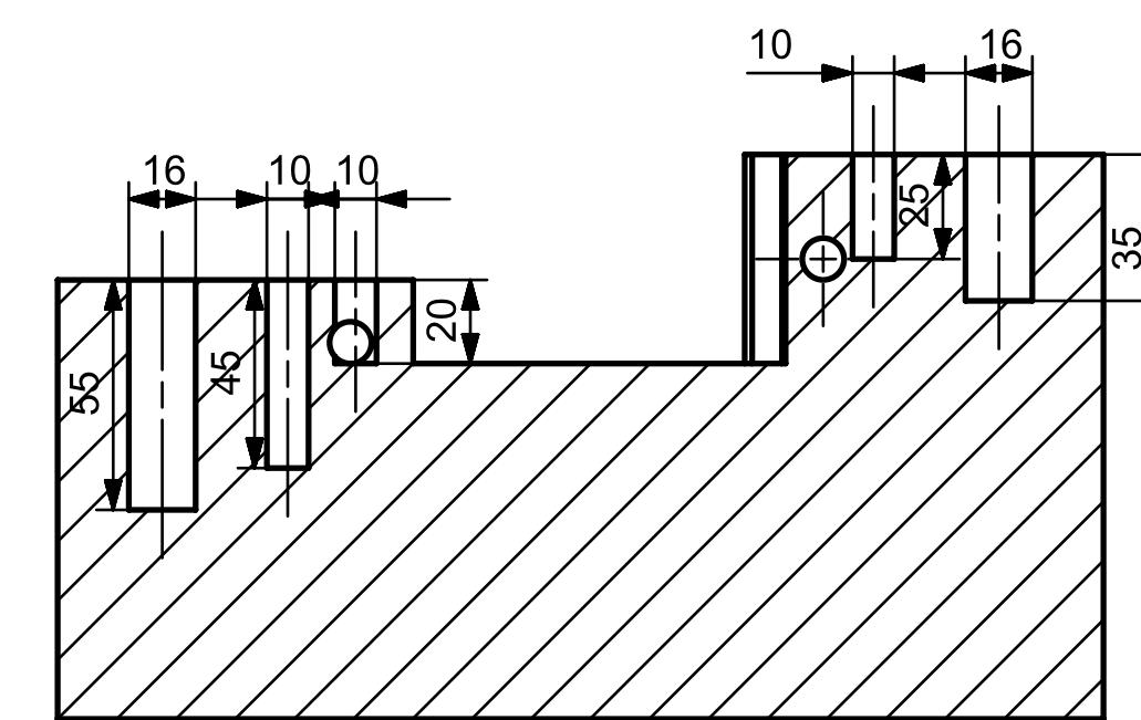
SECTION D-D
