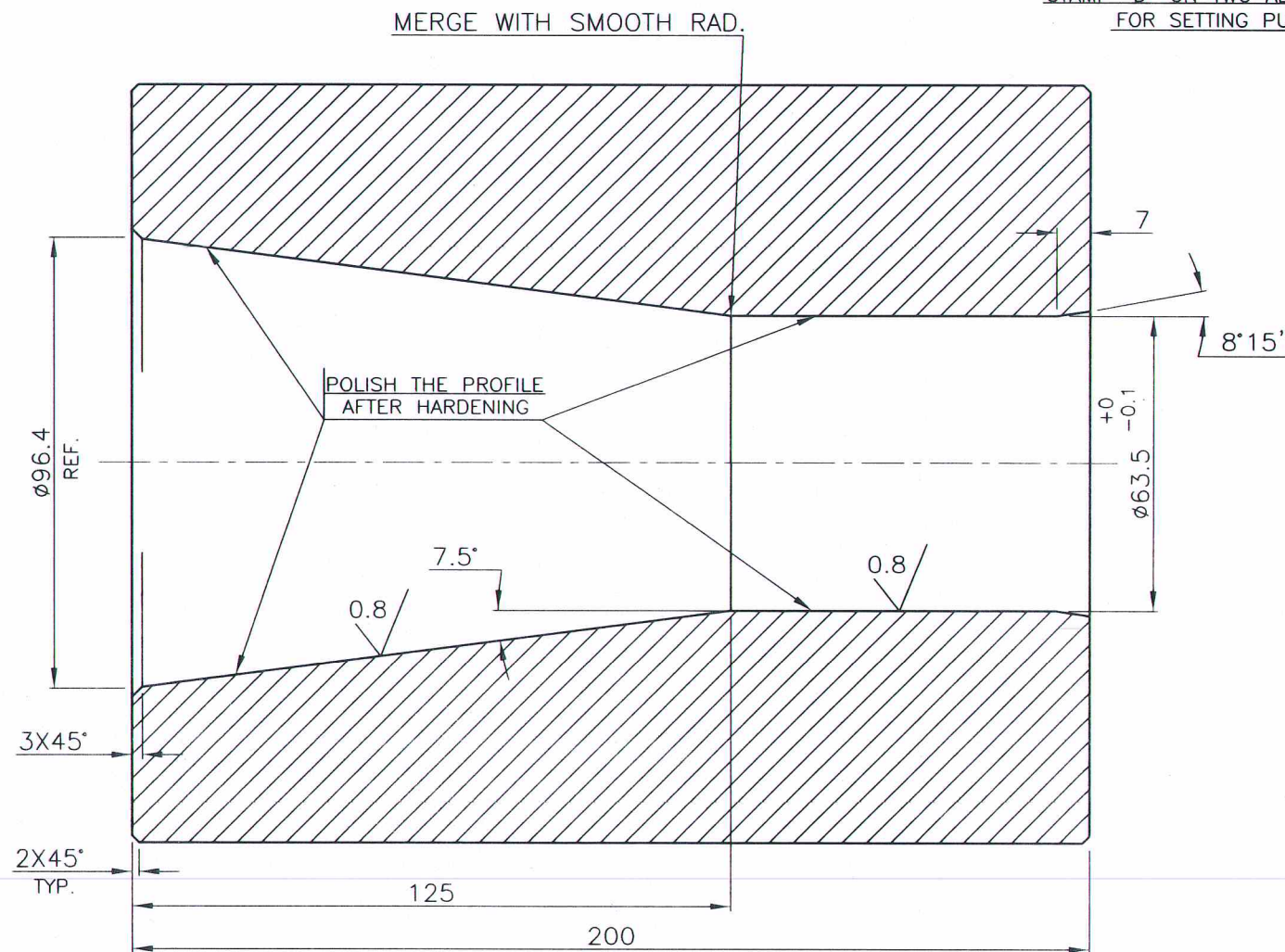
SECTION A-A
