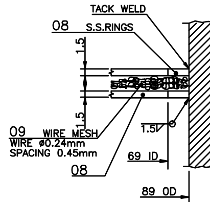
DETAIL : 1
