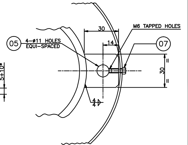
SECTION : 3-3
