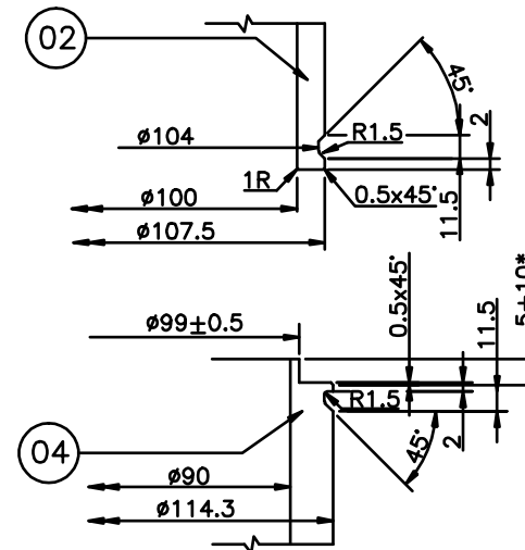
DETAIL : 2
