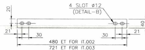
ITEM-002,003
