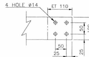
DETAIL-E
