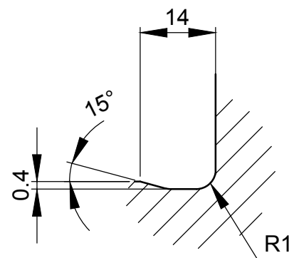
DETAIL - Y
