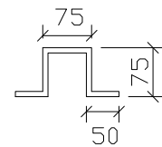
LUG DETAILS
