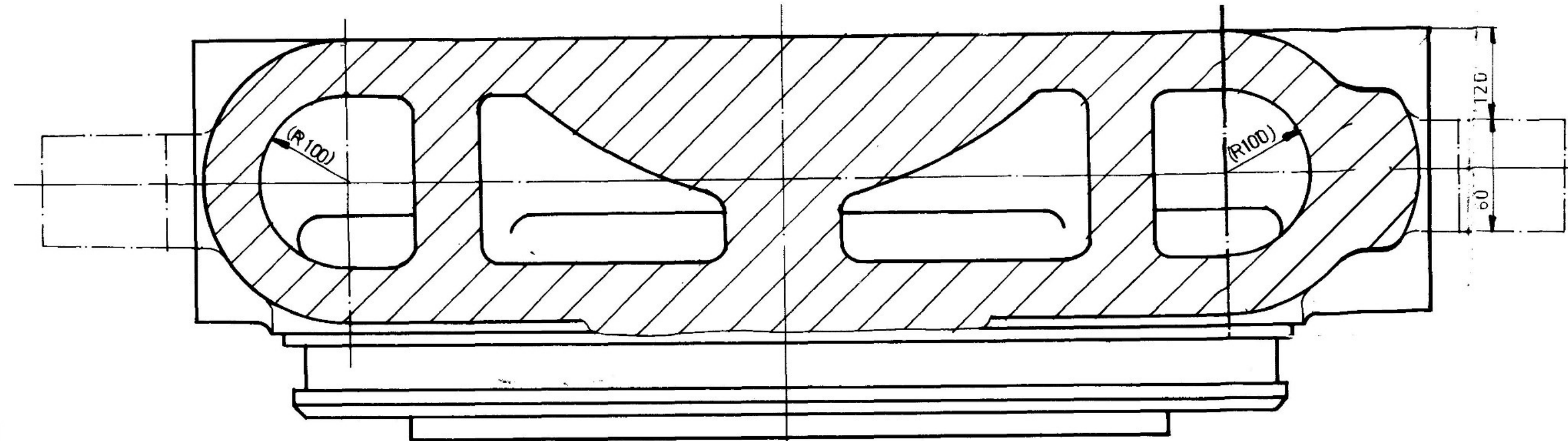
SECTION D-D
