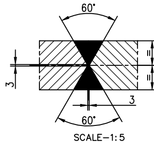
SCALE-1:5
