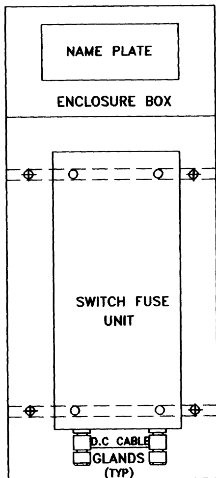
ELEVATION
