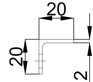
SAG Angle (20LU20x2) SCALE - 20:1
