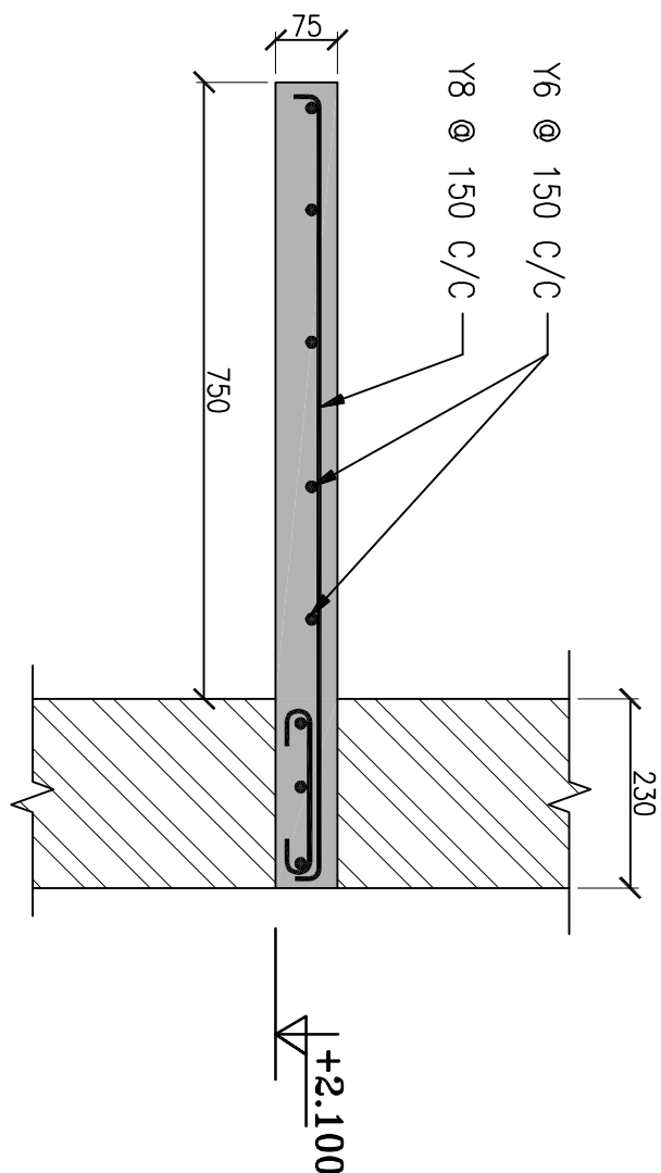
S E C T I O N - A A
