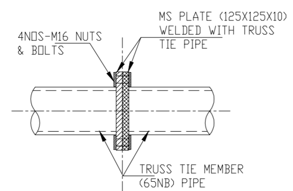
JOINT-2 (TYP.)
