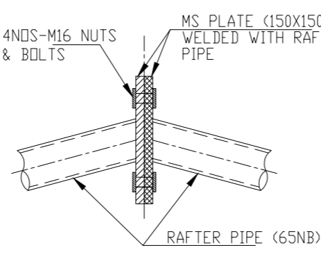
JOINT-3 (TYP.)
