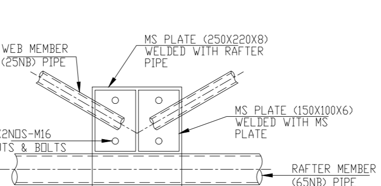
JOINT-6 (TYP.)
