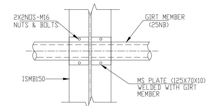
JOINT-4 (TYP.)
