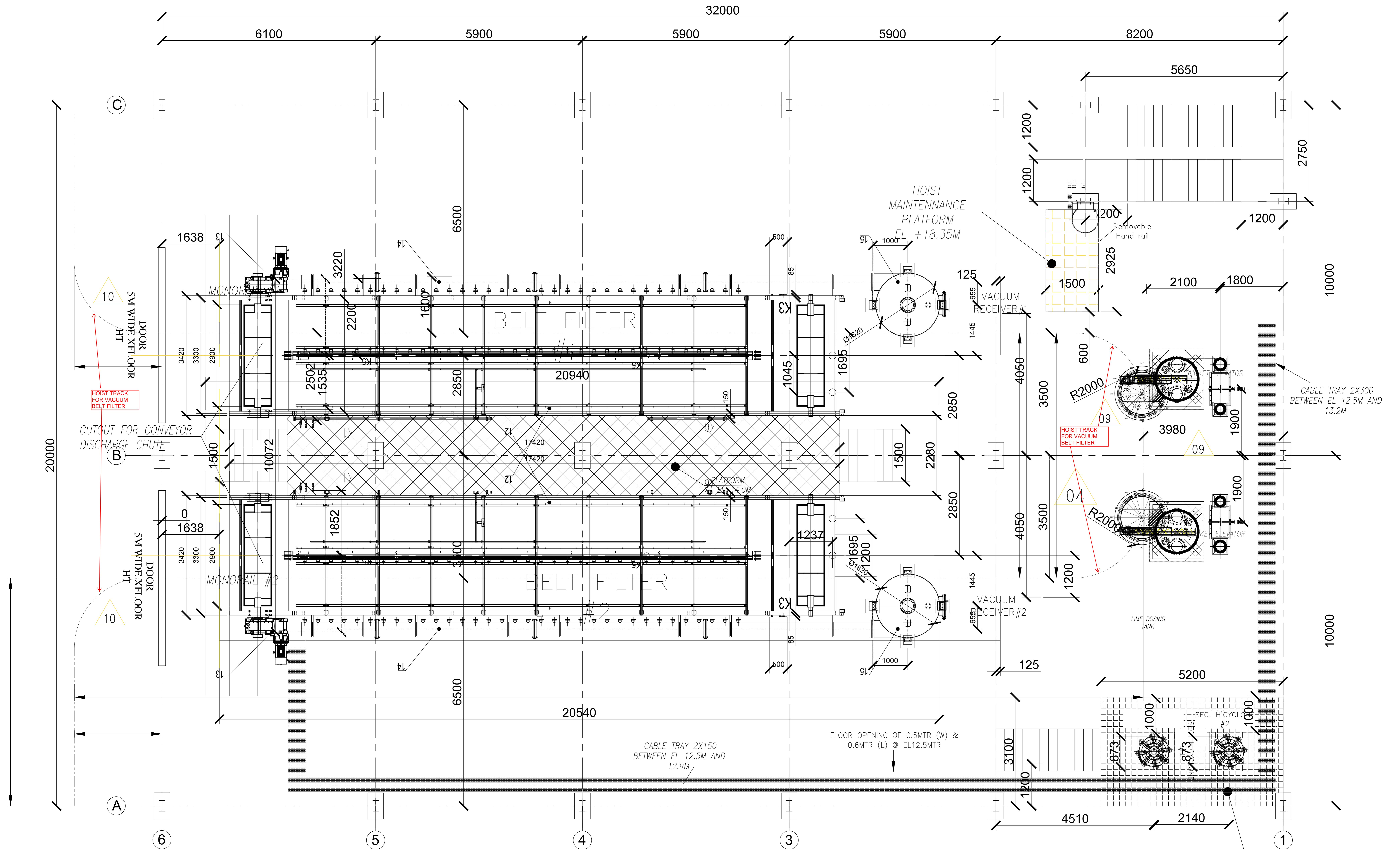
PLAN @ EL +12.5m
