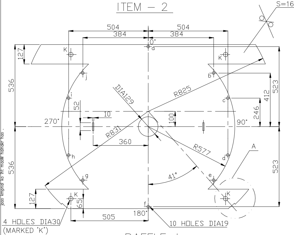
BAFFLE-I (VAR. 01)
