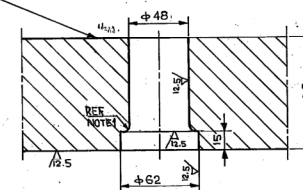
SECTION A-A SCALE 1:2
