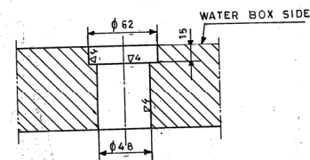
I SCALE 1:2
