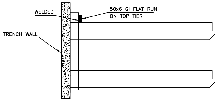
DETAIL 'G'
