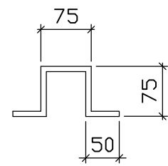
LUG DETAILS
