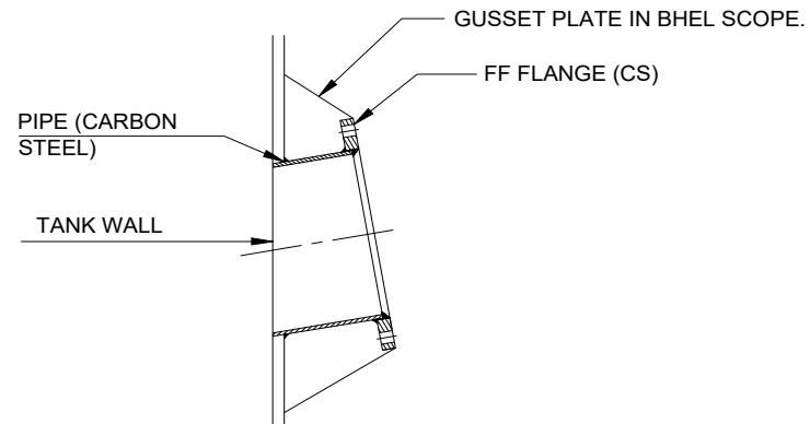
DETAIL-A (AGITATOR NOZZLE)
