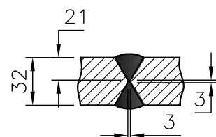
EDGE PREPARATION FOR ITEM-02
