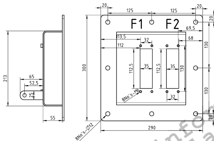
(viii) F1,F2 Coupler Plate – Original
