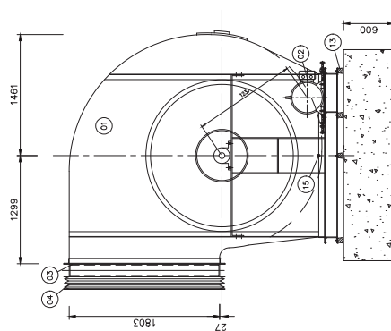
FAN DRIVE END ELEVATION
