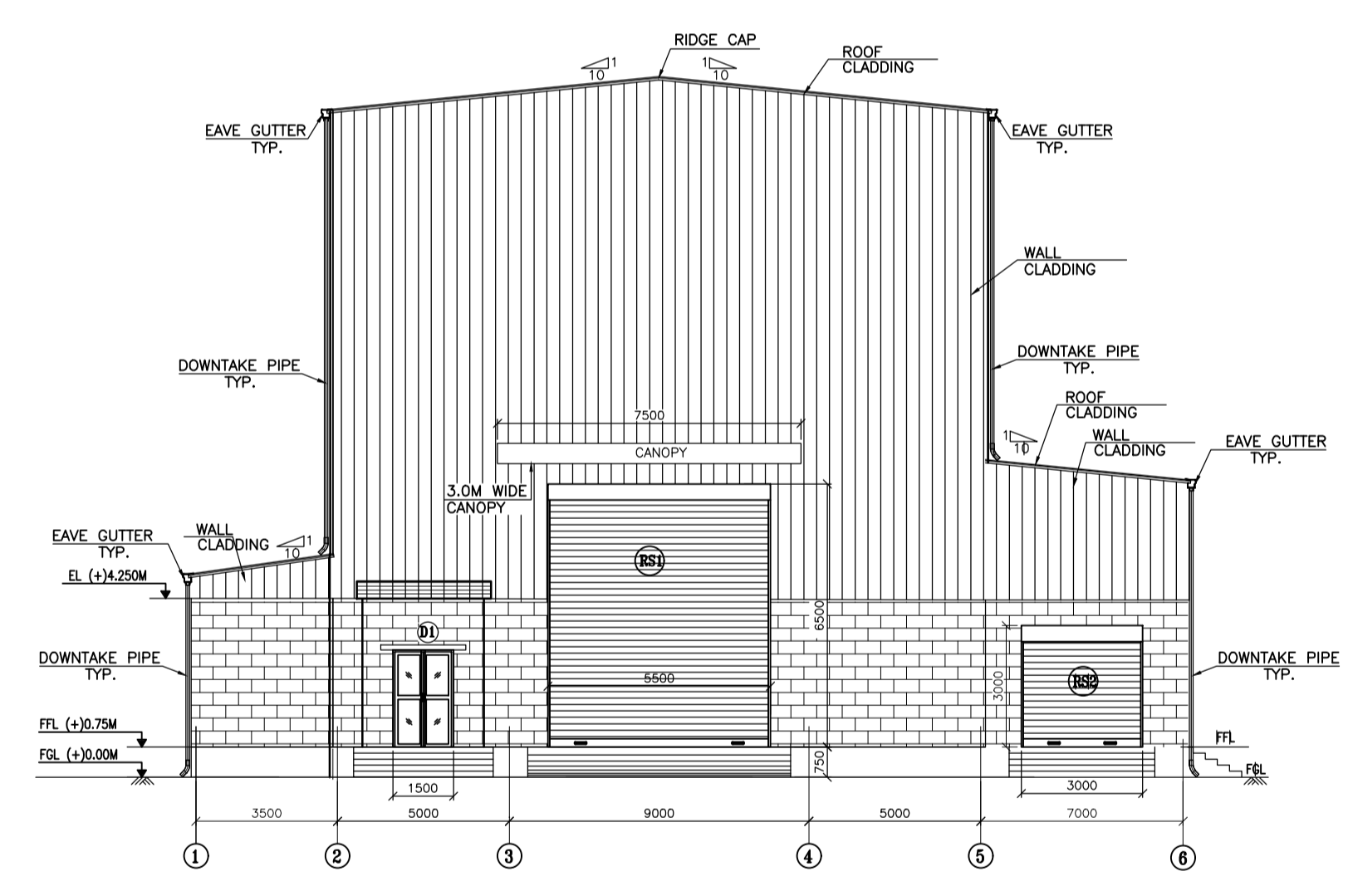
ELEVATION -A
