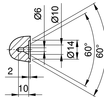
DETAIL - Y
