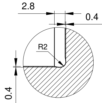
DETAIL - Y SCALE - 1:5
