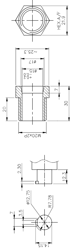
DETAIL-D
