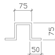
LUG DETAILS
