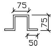
LUG DETAILS
