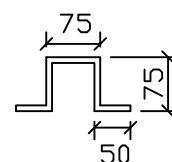
LUG DETAILS
