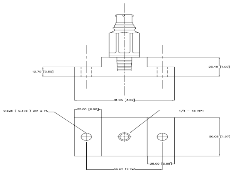
FIG: 2.1.4a: VELOCITY PROBE
