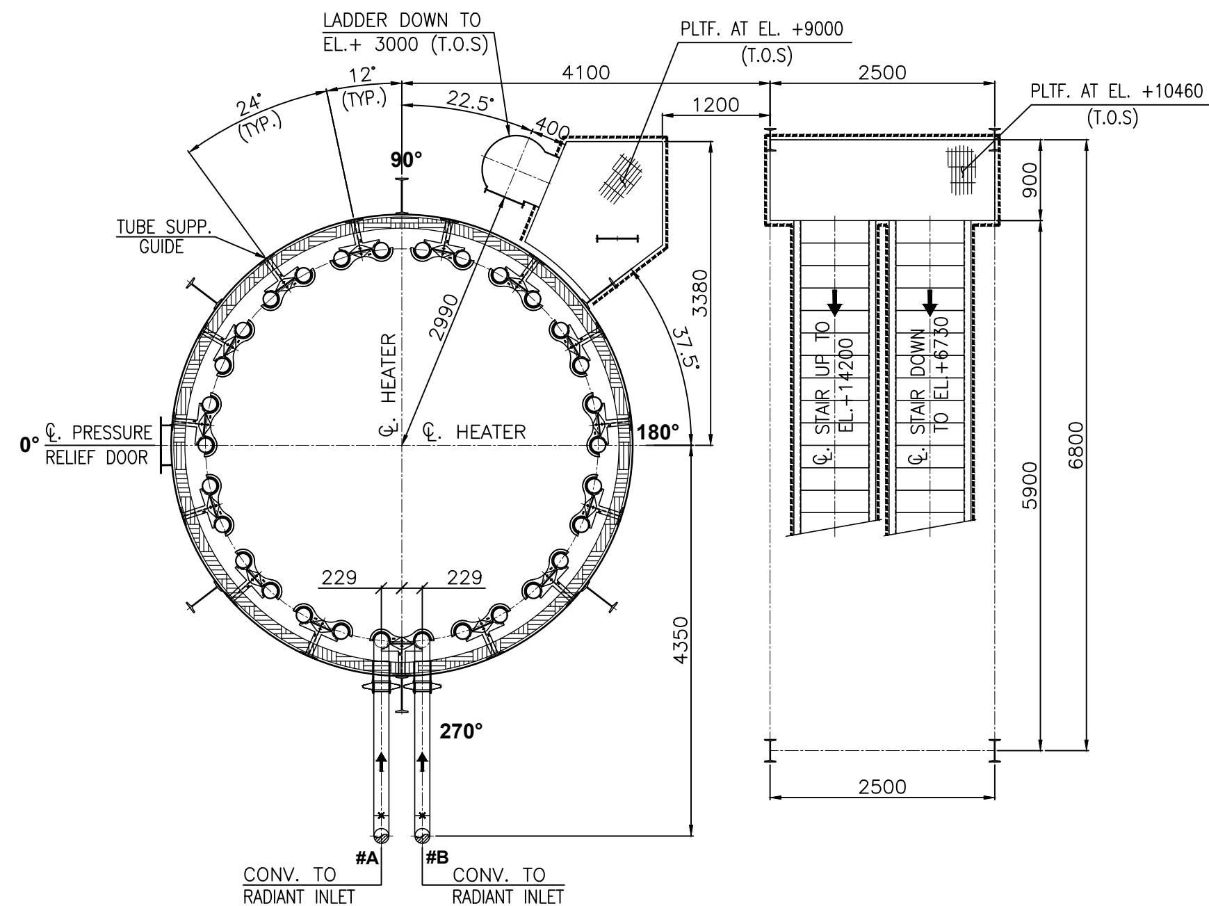
SECTION D-D
