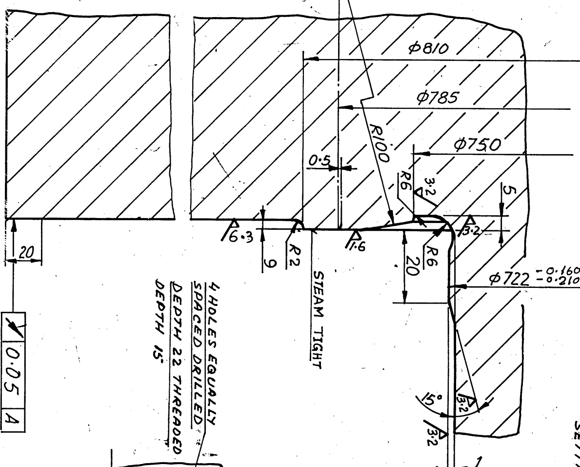
DETAIL II (ZONE-E11)
