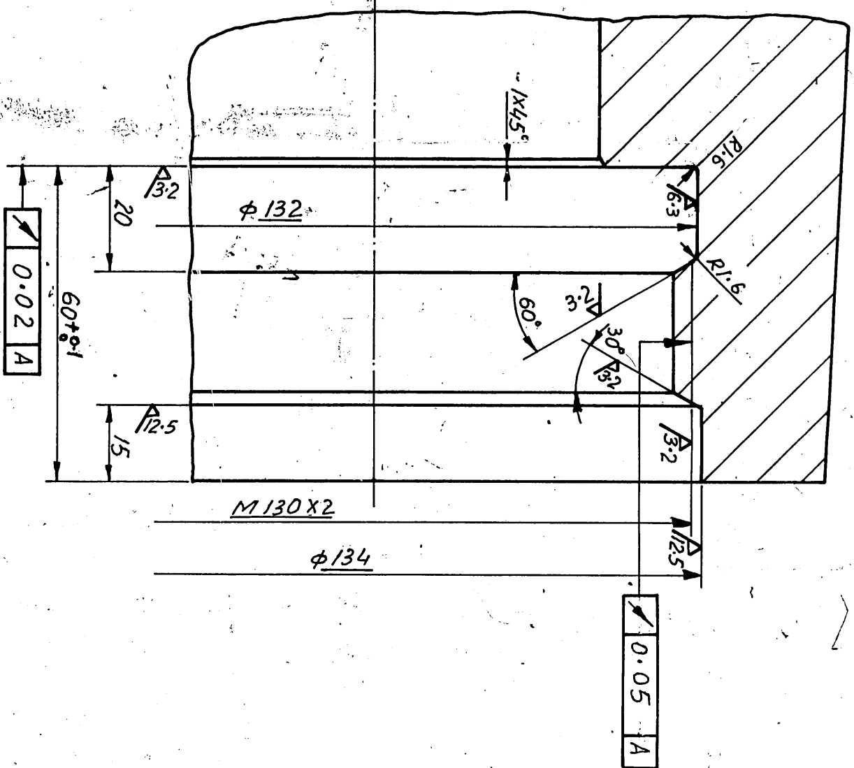
DETAIL-III (ZONE-G-9)
